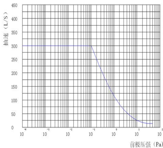
图-2 JTFB-300Z 脂润滑风冷分子泵对空气的压缩比曲线
