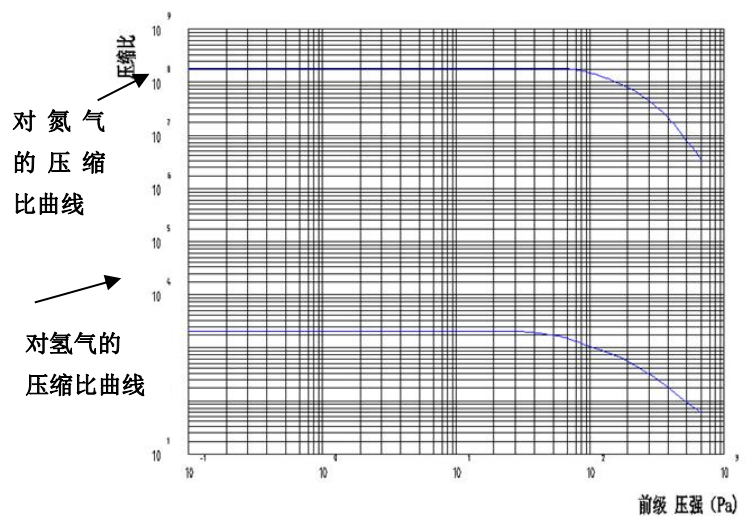
图-3 JTFB-300Z 脂润滑风冷分子泵对氮气及氢气的压缩比曲线
